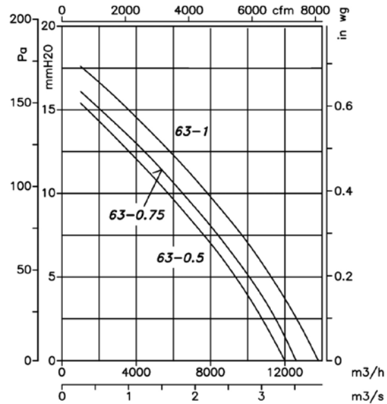
6 Polos=1000 r/min
