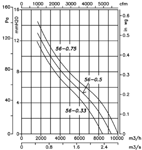
6 Polos=1000 r/min
