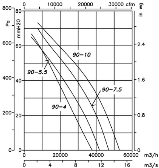
4 Polos=1500 r/min
