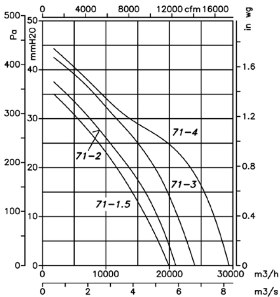
4 Polos=1500 r/min
