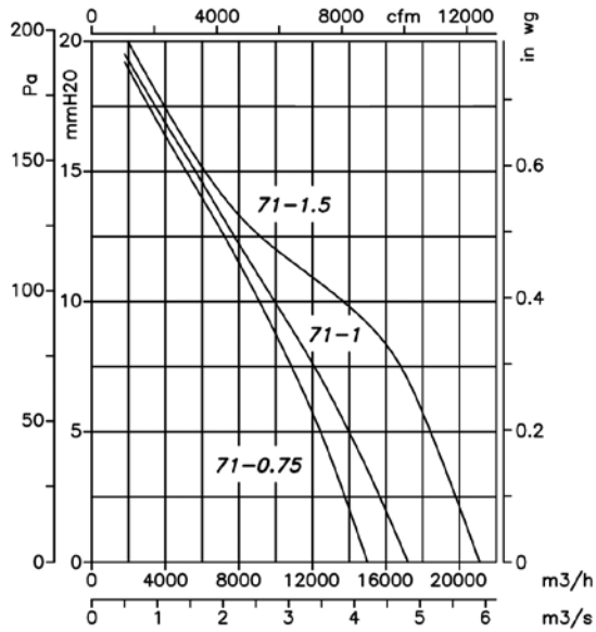
6 Polos=1000 r/min
