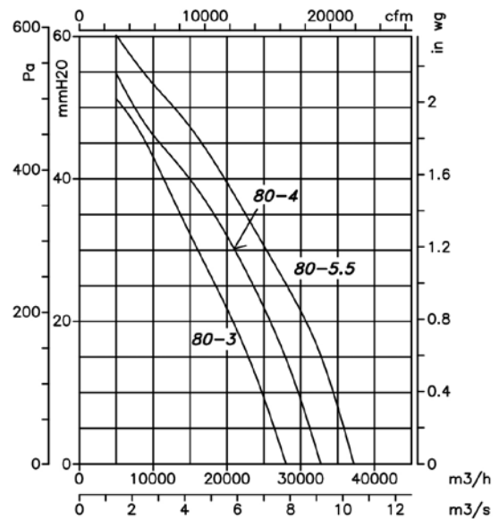
4 Polos=1500 r/min
