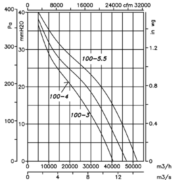
6 Polos=1000 r/min
