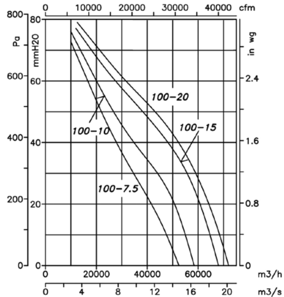
4 Polos=1500 r/min
