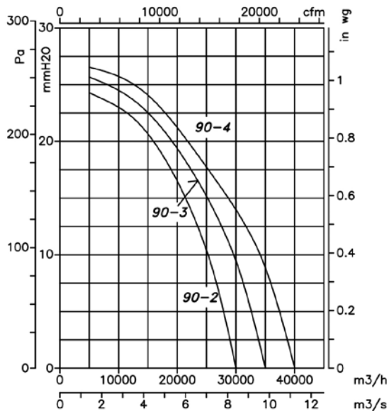
6 Polos=1000 r/min
